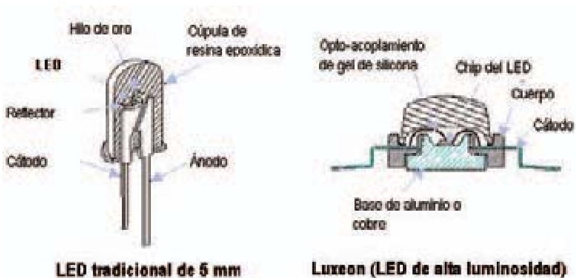
Figura 1 Esquema de LED tradicional y de alta luminosidad.
