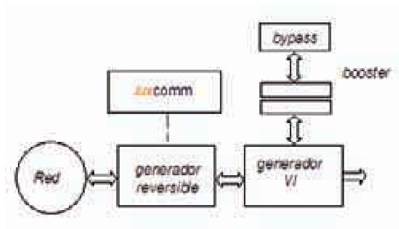
Figura 1 Arquitectura de un Regulador de Flujo Luminosos de elementos electrónicos activos, serie SET-LUX de Zigor.
