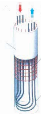
Figura A1.4. Pilote termoactivo. (Fuente: Geoter).
