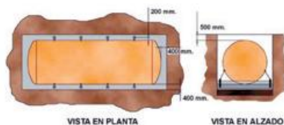
Foto 9. Instalación de un depósito enterrado.
