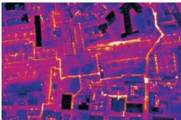
Imagen 23. Termografía aplicada a District Heating. Fuente: Horuslab .
