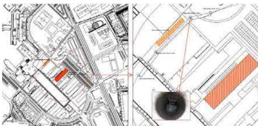
Figura 34. Ubicación del nuevo edificio del CICFANO en el Campus de la Universidad de Aveiro y situación respecto al colector general de aguas residuales que atraviesa el Campus, frente al Rectorado a escasos 70 m del nuevo edificio. Emplazamiento del área donde se va a realizar el by-pass para el intercambiador de energía y pozos de conexión. Fuente: ENERES/KASAG.
