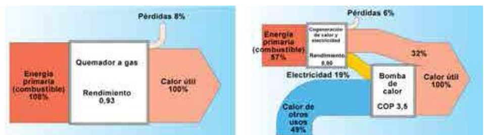
Figura 18. Comparación de la eficiencia energética. Para producir la misma cantidad de calor (energía útil), una instalación de aguas residuales de recuperación de calor, con bomba el calor y producción combinada de calor y electricidad consume dos veces menos energía fósil que un sistema convencional. Fuente: ENERES/KASAG.
