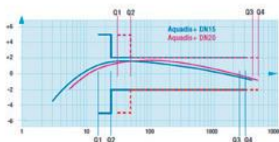
Figura 10. Contador clase D y curva de error.
