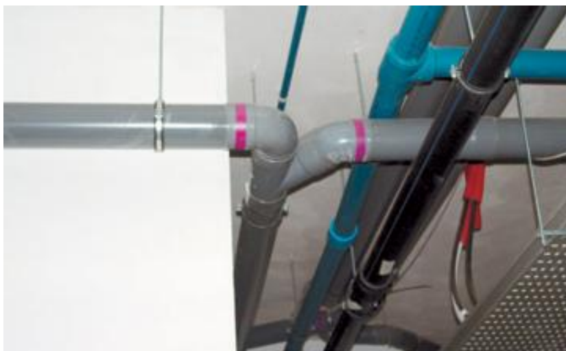
Foto 5. Red de evacuación de aguas grises señalizada.
