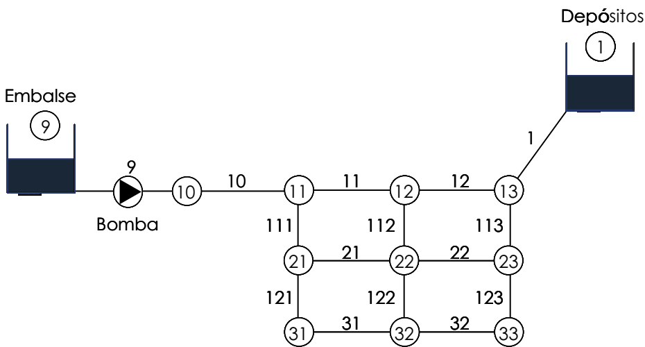
Figura 2. Esquema de la red
