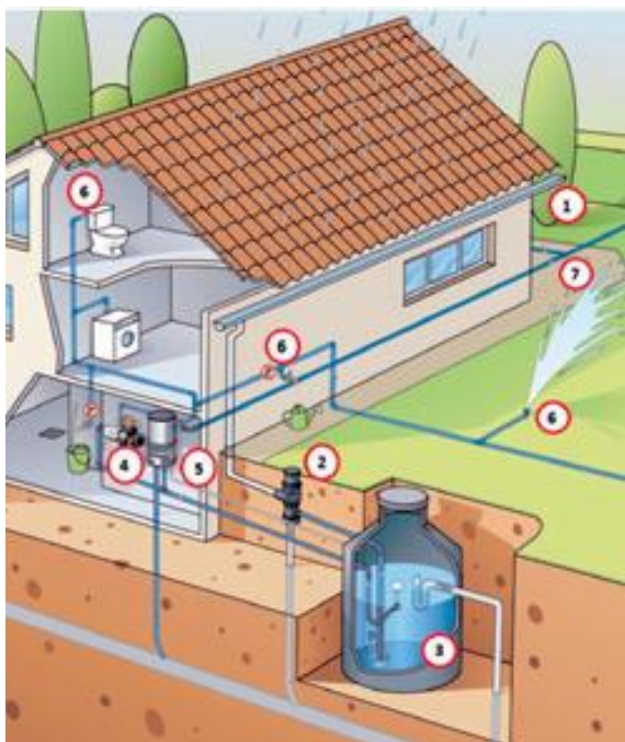
Figura 8. Ejemplo gráfico de una instalación para el aprovechamiento de aguas de lluvia controlada por módulo de automatización.
