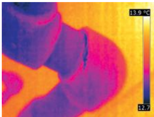
Imagen 17. Localización de una pequeña rotura en la red de PPR del agua fría sanitaria.
