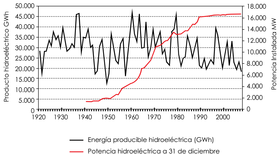
Figura 2. Producible hidroeléctrico vs. Potencia instalada. Fuente: Red Eléctrica Española, www.ree.es
