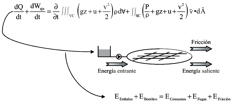
Figura 6. Planteamiento conceptual de la auditoría energética de una red y sus ecuaciones principales
