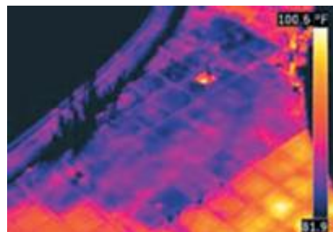
Imagen 18. En piscinas como la de la imagen, donde se observa la presencia de agua en una zona. Además, en piscinas climatizadas también es útil para determinar el grado de estanqueidad del cerramiento. Fuente: Flir Systems.
