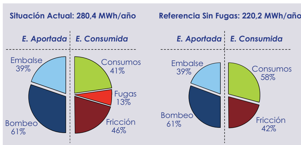
Figura 7. Resultados de la auditoría energética de la red
