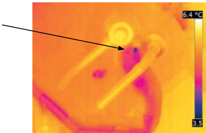
Imagen 2. Termograma de la bajante.
