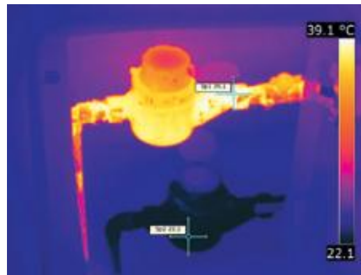
Imagen 13. En los contadores de las viviendas se encuentra sin aislar el del agua ca-liente, con un importante efecto radiador de calor.
