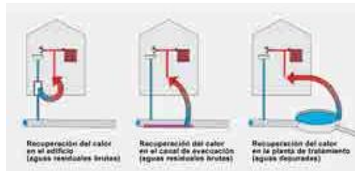
Figura12. Potenciales emplazamientos de la instalación de recuperación e intercambio de calor en la red de recogida u tratamiento de aguas residuales. Fuente: ENERES/KASAG.
