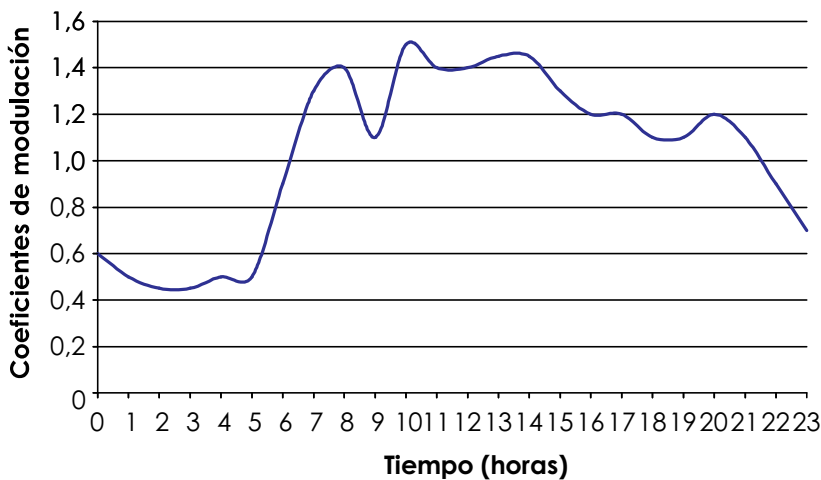
Figura 3. Modulación de los consumos
