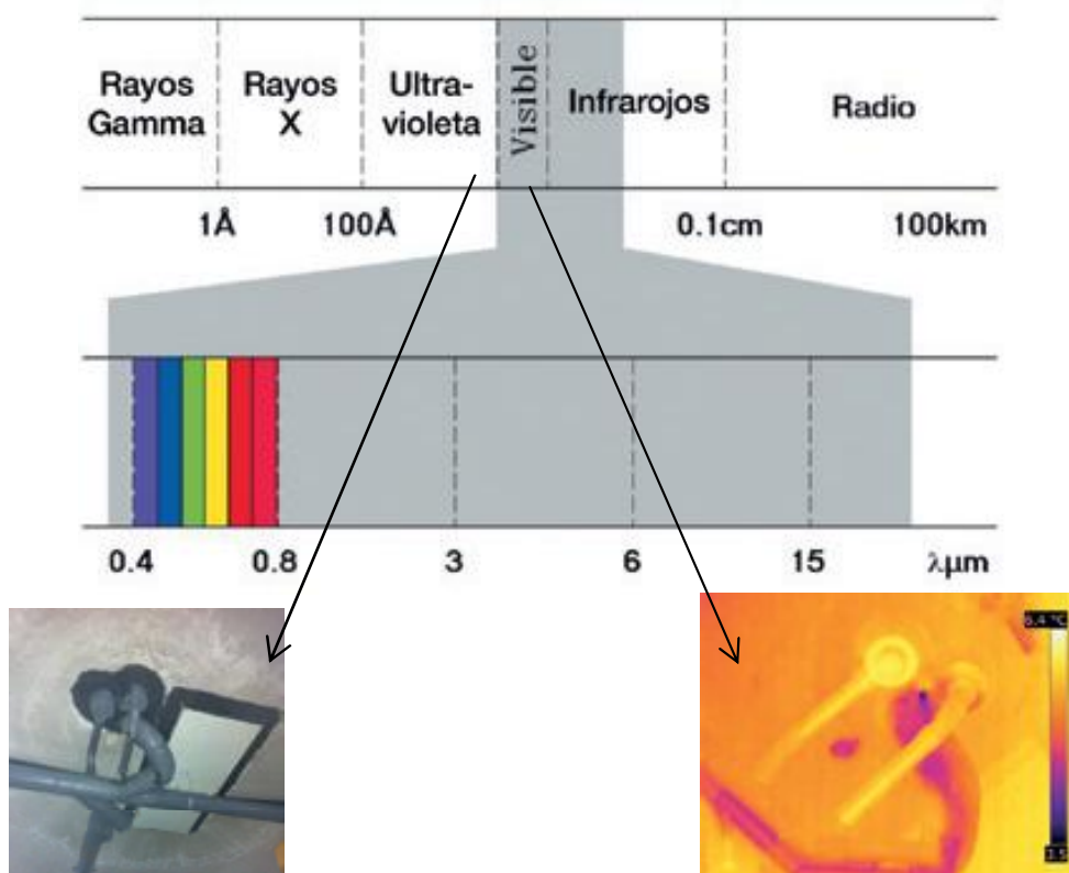
Figura 2. Espectro electromagnético (eBuilding).
