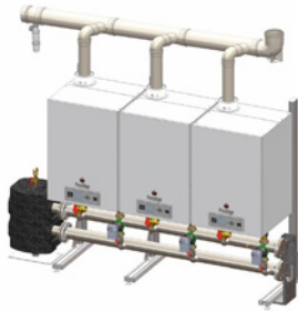
Ejemplo de instalación de calderas murales en cascada
