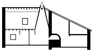
Sección típica de casa de la Sierra del Rincón. Horno colgante Montejo de la Sierra
