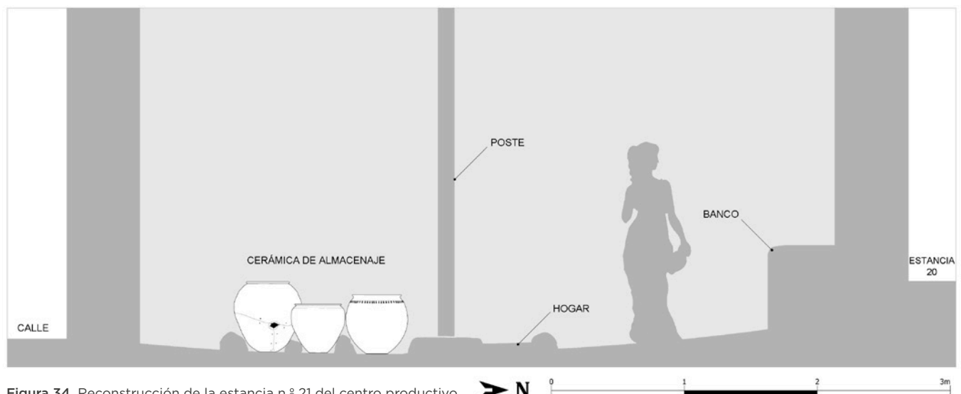
Figura 34. Reconstrucción de la estancia n.º 21 del centro productivo.
