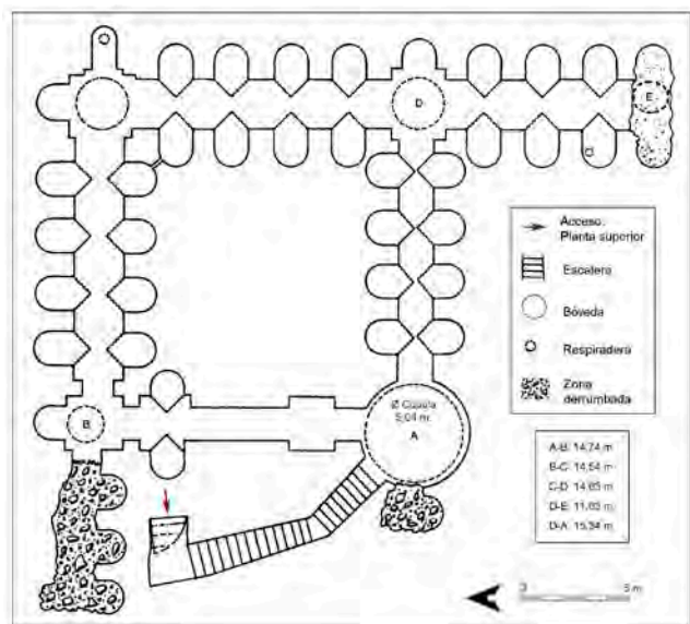
Figura 150. Planimetría de la Cueva de la Luna (tomada de Rico, 1984, y modificada por Carmen Valenciano Prieto).
