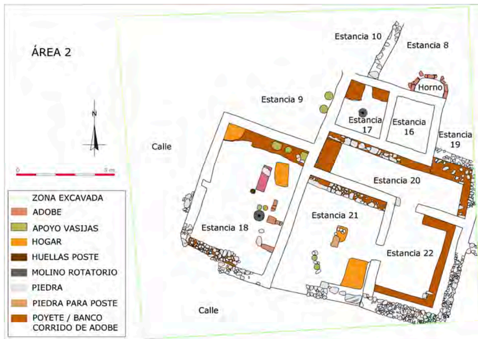
Figura 29. Plano del centro productivo. Fase III (Área 2).
